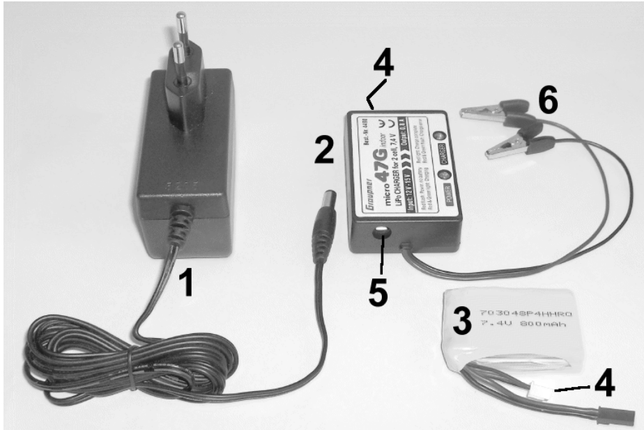
Fig.6 : Charge de l'accu LiPo: 1. Transformateur de courant secteur – 2. Chargeur – 3. Accu LiPo - 4. Prises de charger – 5. Prise d'entrée – 6. Pinces crocodile.
