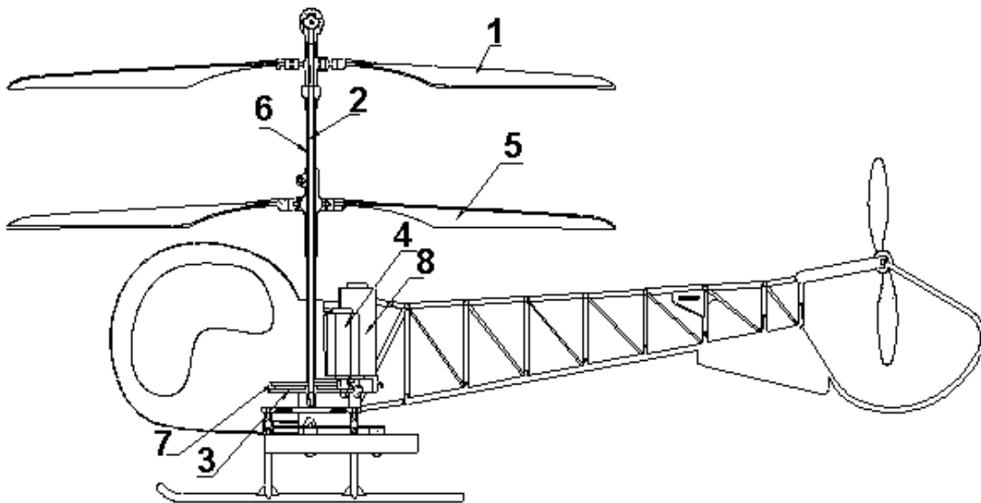
Fig.1 : Disposition schématique du système de rotors coaxiaux 1. Pale de rotor supérieur – 2. Arbre intérieur de rotor - 3. Réducteur du rotor supérieur – 4. Moteur du rotor supérieur – 5. Pale de rotor inférieur – 6. Arbre extérieur de rotor – 7. Réducteur du rotor inférieur – 8. Moteur du rotor inférieur.
