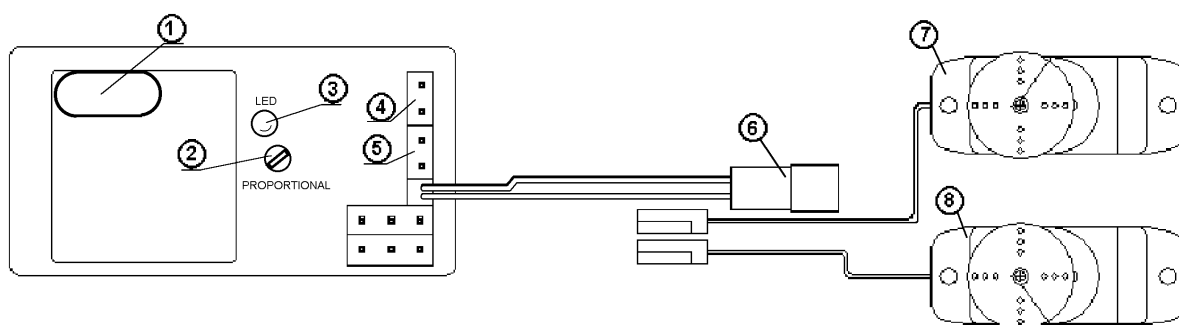
Fig.3 : Câblage de l'électronique de bord "4 en 1"
