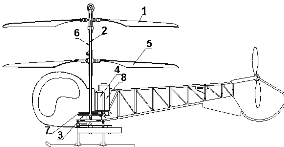
Abb. (1): Schematische Anordnung des Koaxialrotorsystems
