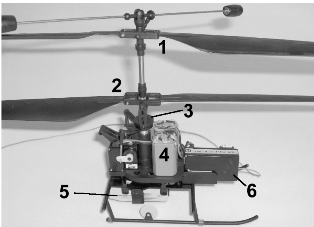
Abb. (5): Rechte Seite des Hubschraubers: 1. Oberer Rotor 2. Unterer Rotor 3. Taumelscheibe 4. Motoren 5. Servos 6. "4 in 1" - Bordelektronik
